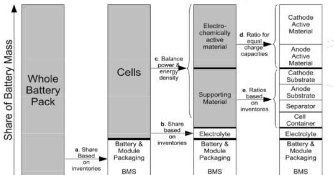
Figure 8-1 Exemple de décomposition d'une batterie
