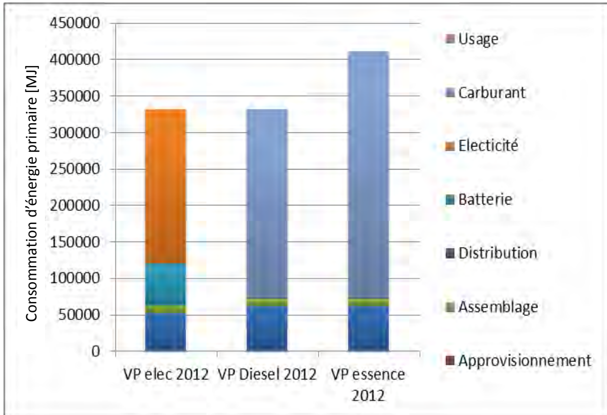
Figure 4-1 Contribution à la consommation d'énergie primaire des différentes étapes du cycle de vie des véhicules particulier électrique, Diesel et essence à l'horizon 2012.
