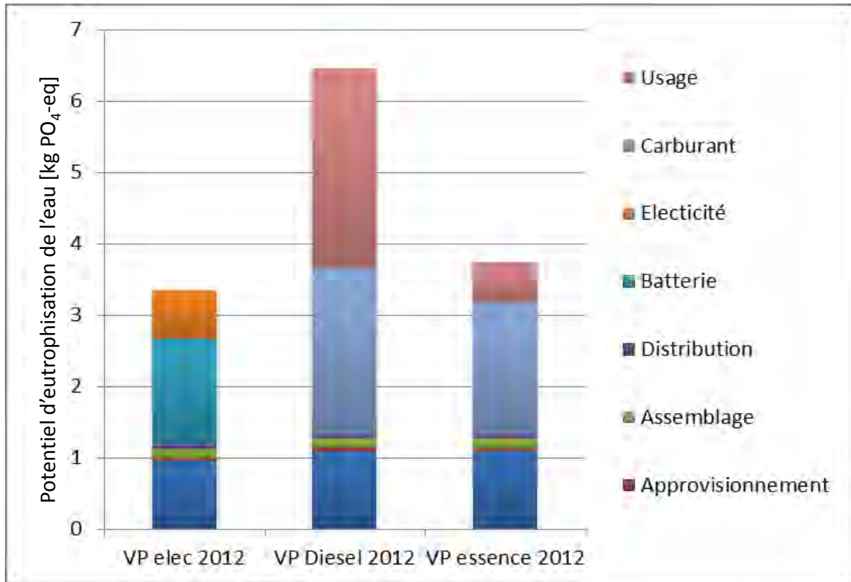
Figure 4-6 Contribution au potentiel d'eutrophisation des différentes étapes du cycle de vie des véhicules particuliers électrique, Diesel et essence à l'horizon 2012.
