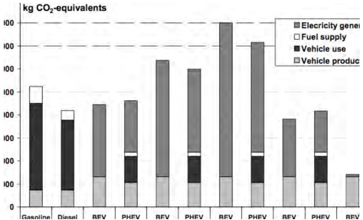
Figure 8-2 Emissions GES du cycle de vie d'un véhicule compact avec différents groupes motopulseurs (120 000 km, 70% route de ville)
