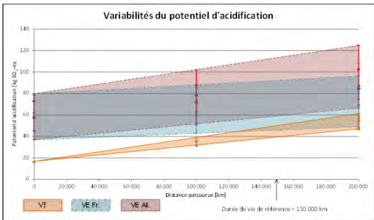
Figure 4-67 Variabilité du potentiel d'acidification du cycle de vie complet (sans le scénario de fin de vie)
