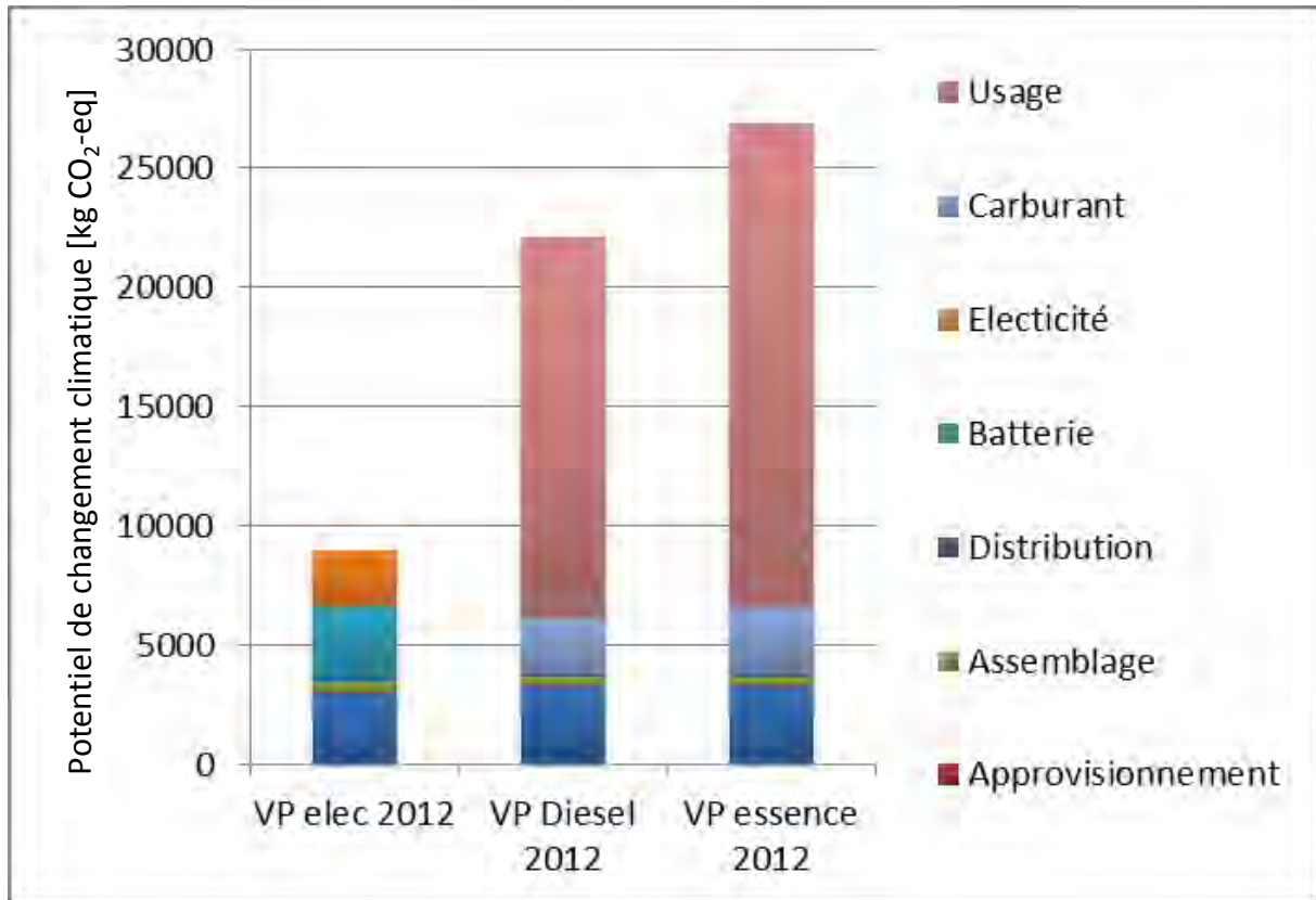
Figure 4-2 Contribution au potentiel de changement climatique des différentes étapes du cycle de vie des véhicules particuliers électrique, Diesel et essence à l'horizon 2012.
