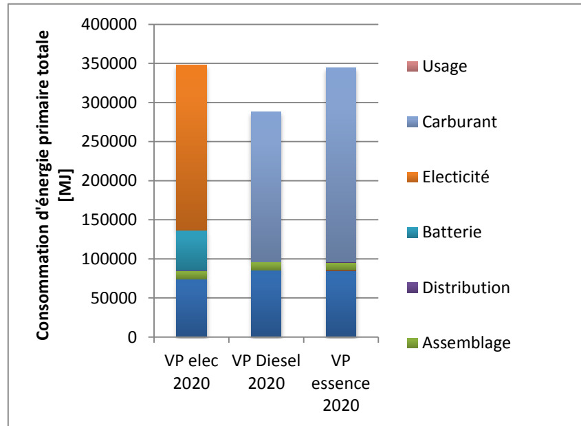
Figure 4-12 Contribution à la consommation d'énergie primaire des différentes étapes du cycle de vie des véhicules particulier électrique, Diesel et essence à l'horizon 2020.
