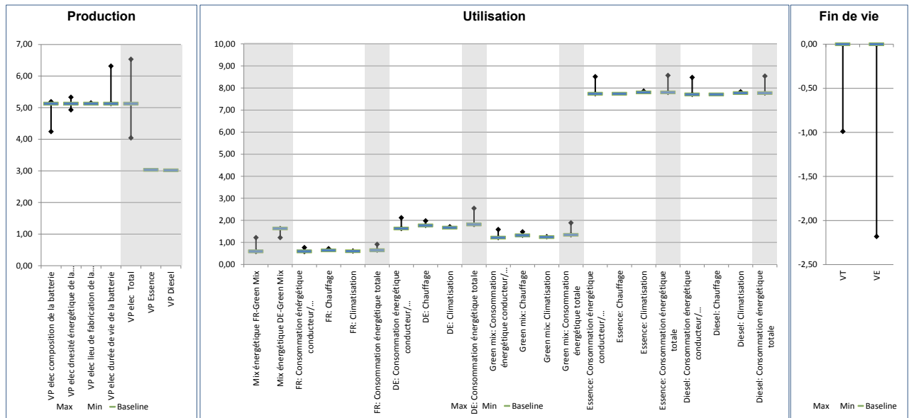
Figure 4-70 Incertitudes pour le potentiel de création d'ozone photochimique pour la production, l'utilisation et la fin de vie
