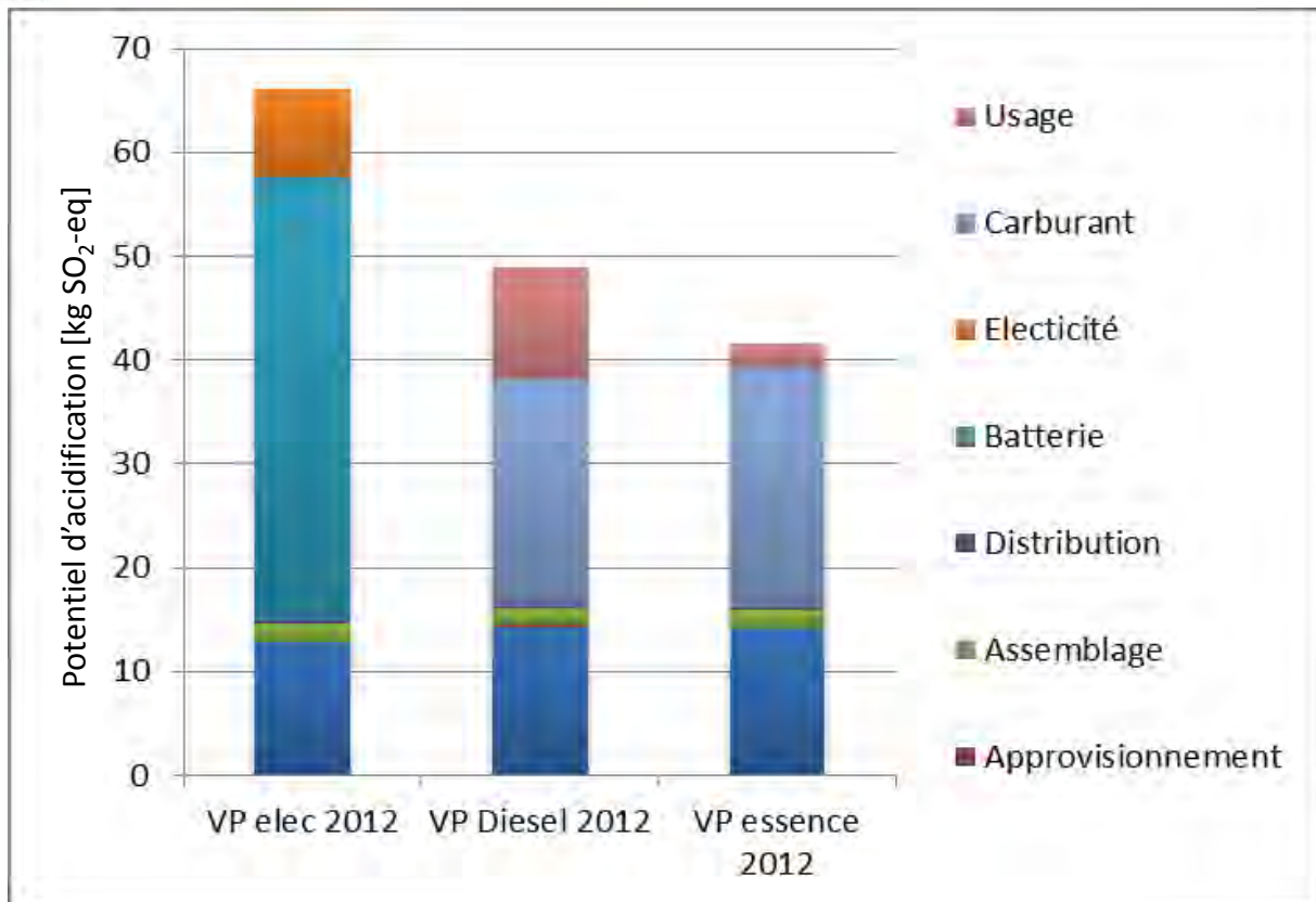
Figure 4-5 Contribution au potentiel d'acidification des différentes étapes du cycle de vie des véhicules particuliers électrique, Diesel et essence à l'horizon 2012.
